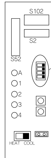
Сервисная Р-плата
