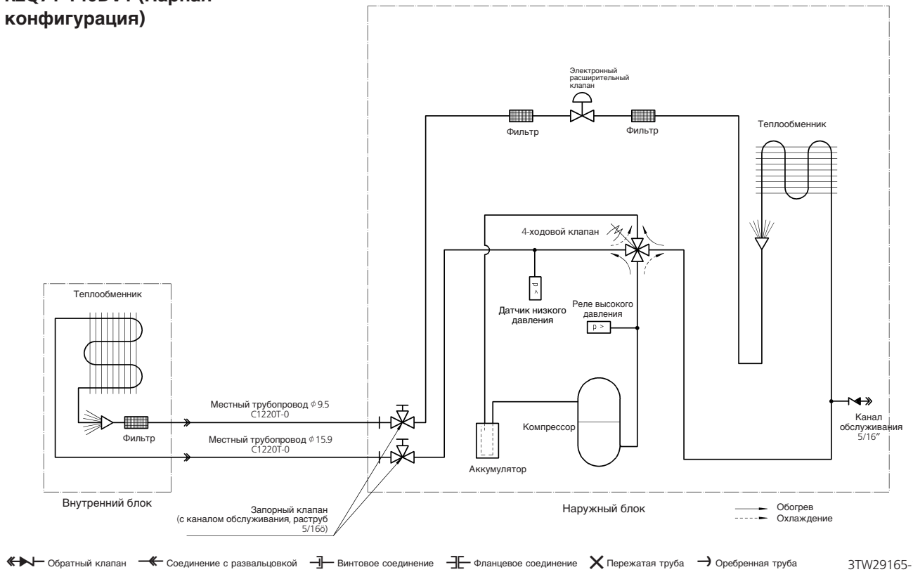
RZQ71-140DV1 (Двухблочная конфигурация)
