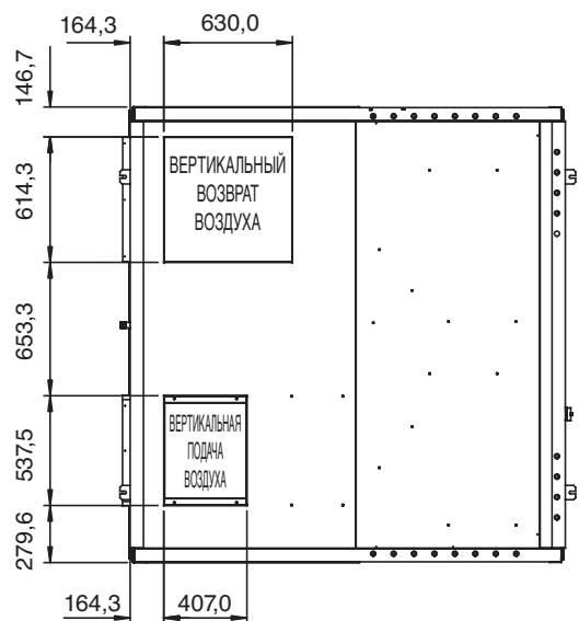
ДЛЯ ВЕРТИКАЛЬНОГО ВЫПУСКА
