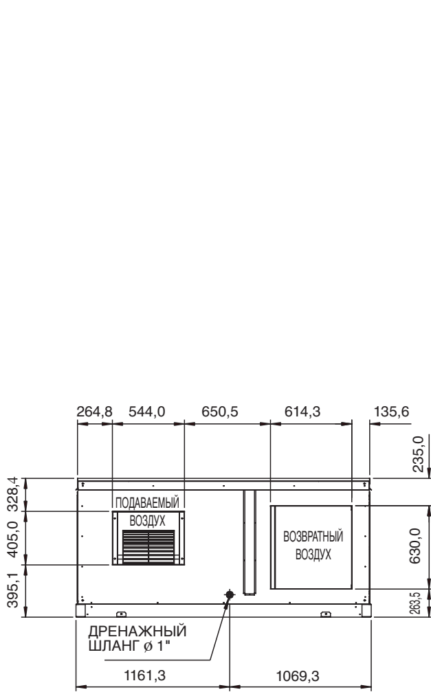
ДЛЯ ГОРИЗОНТАЛЬНОГО ВЫПУСКА
