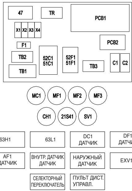
СХЕМА РАСПОЛОЖЕНИЯ
