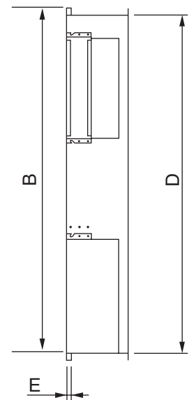
Секция В-В
