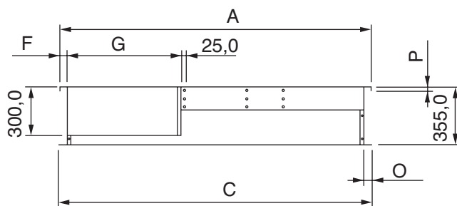
Секция С-С
