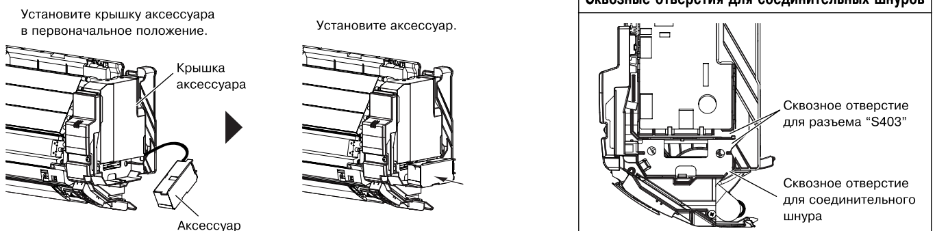
Рисунок 3: Установка аксессуара
