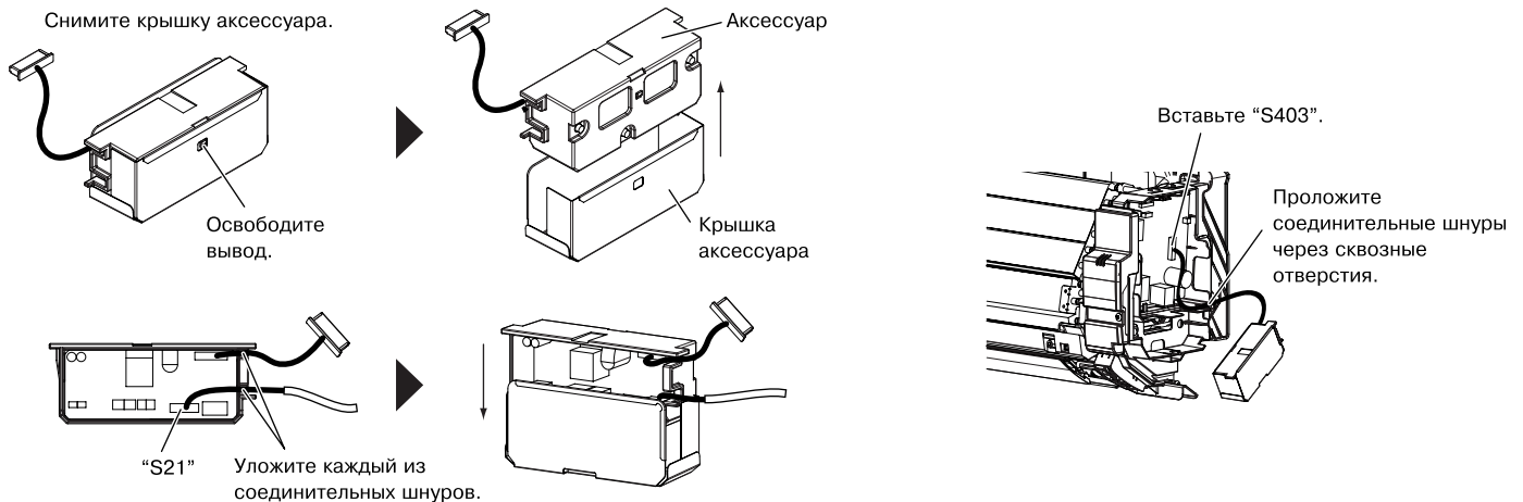
Рисунок 2: Подготовка аксессуара
