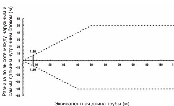
Поправочный коэффициент для производительности по отоплению
