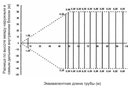
Поправочный коэффициент для производительности по отоплению
