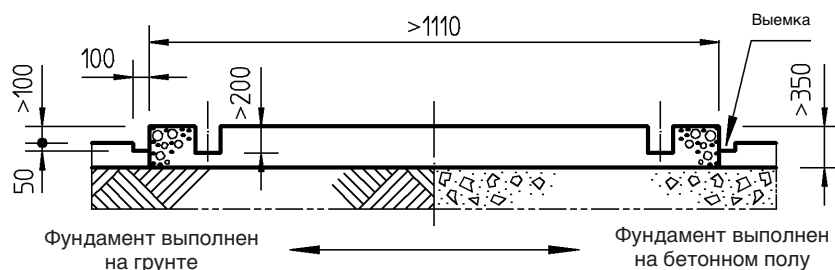
Разрез X-X
