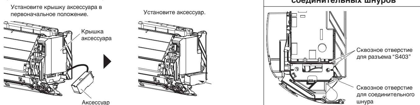
Рисунок 3: Установка аксессуара
