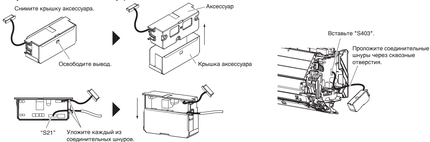
Рисунок 2: Подготовка аксессуара
