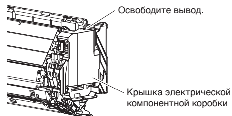
Рисунок 1: Снятие крышки с электрической компонентной коробки
