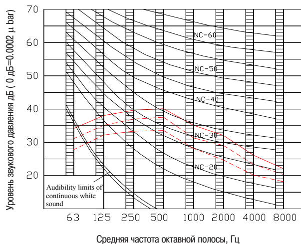
КТНХ50(60,72)НFAN1
