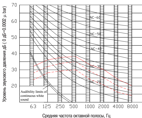
КТНХ40НFAN1
