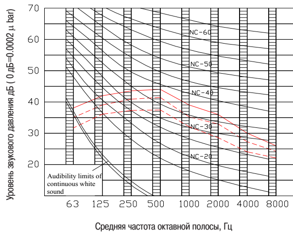
КТНХ115(140)НFAN1
