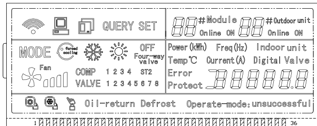
Схема 2 – ЖК-дисплей
