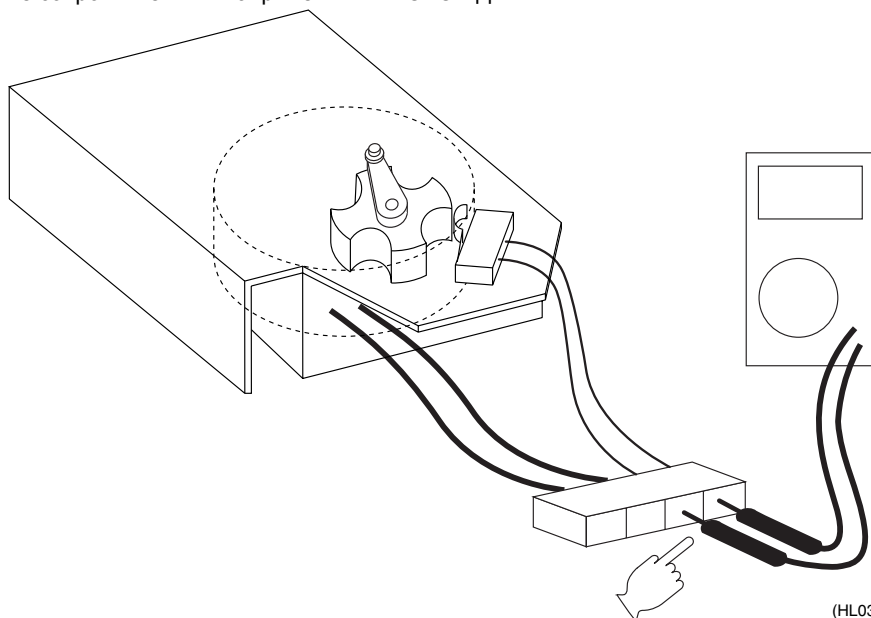
Измерение сопротивления и напряжения — МОТОР ДЕМПФЕРА
