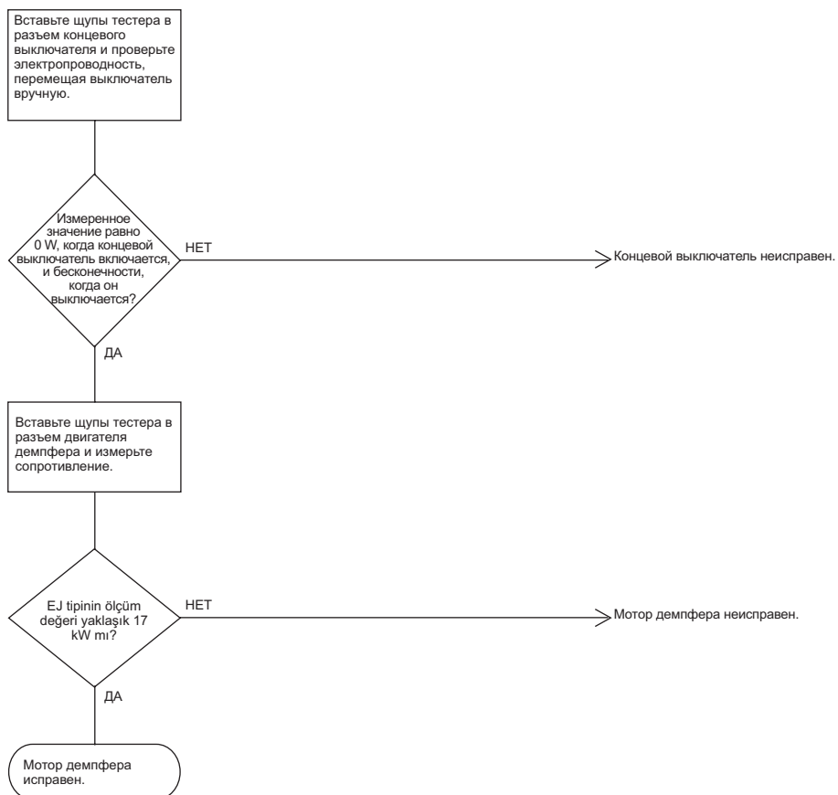
Измерение сопротивления и напряжения — МОТОР ДЕМПФЕРА
