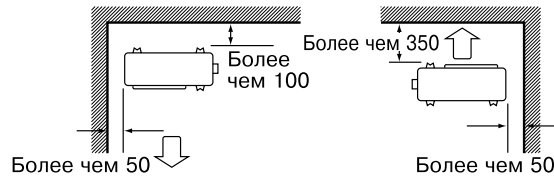
Вид сверху
